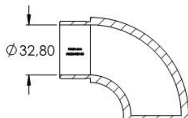
SCHNITT A-A
