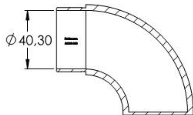
SCHNITT A-A
