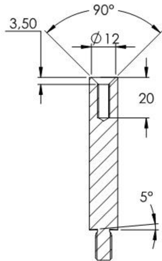
SCHNITT A-A
