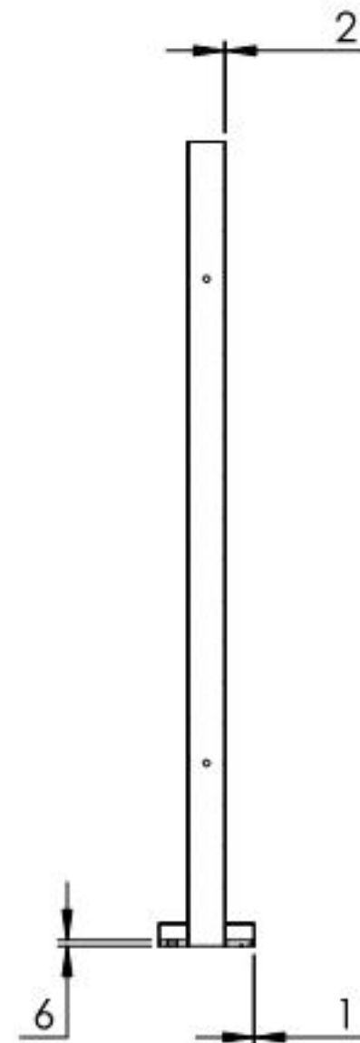
SCHNITT A-A
