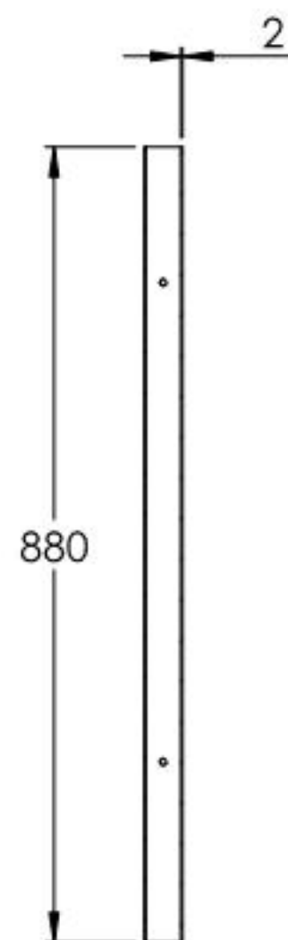
SCHNITT B-B
