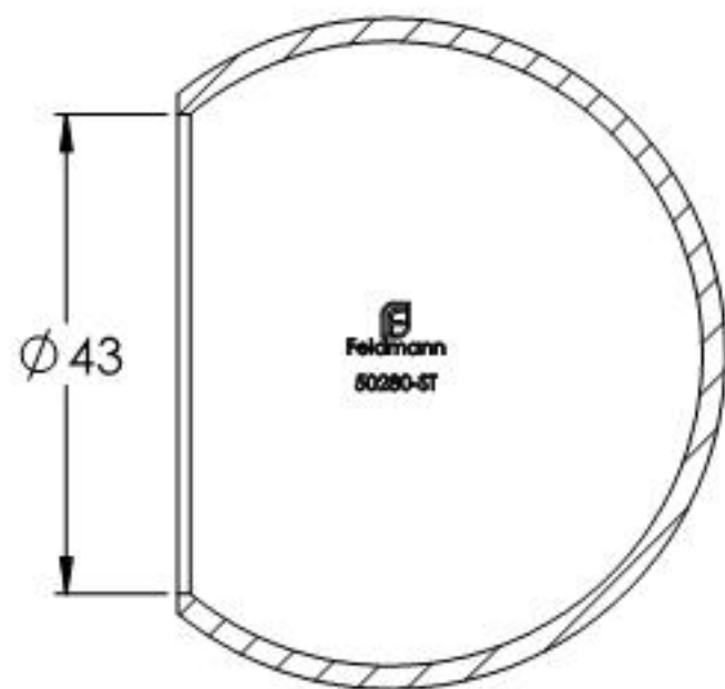
SCHNITT A-A
