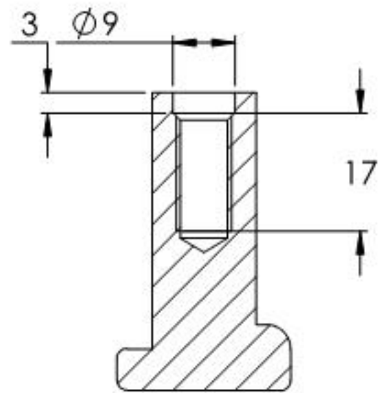
SCHNITT B-B
