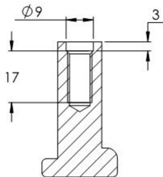
SCHNITT B-B
