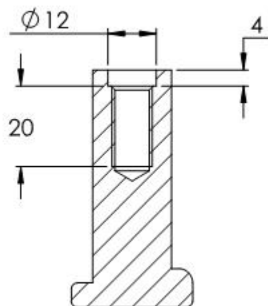
SCHNITT B-B
