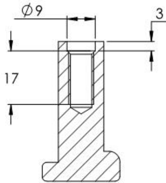
SCHNITT B-B
