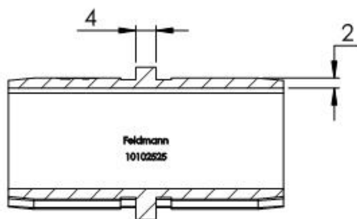
SCHNITT A-A
