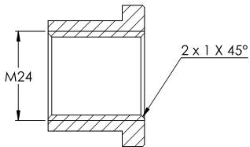
SCHNITT A-A
