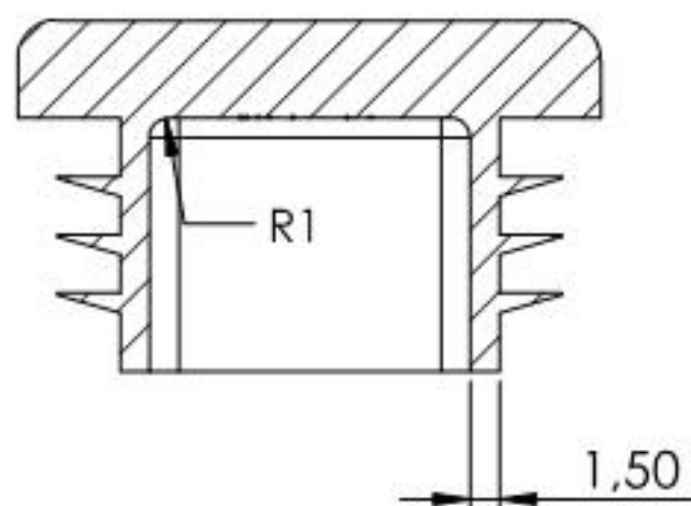
SCHNITT A-A
