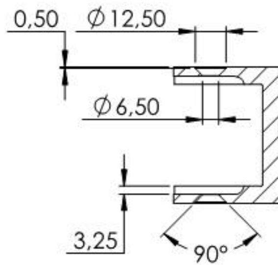
SCHNITT A-A
