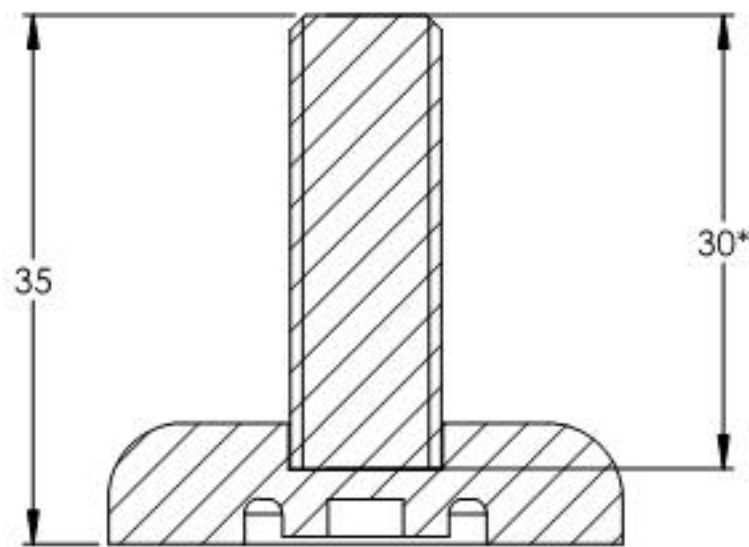
SCHNITT A-A
