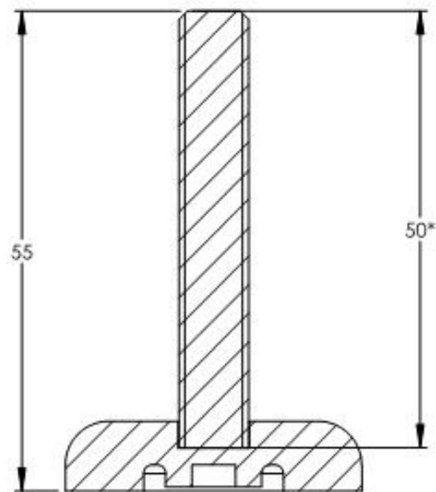
SCHNITT A-A
