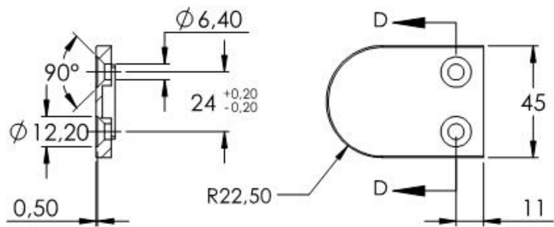
SCHNITT D-D
