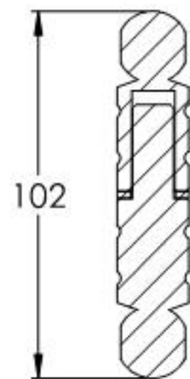
SCHNITT A-A
