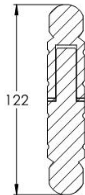
SCHNITT A-A
