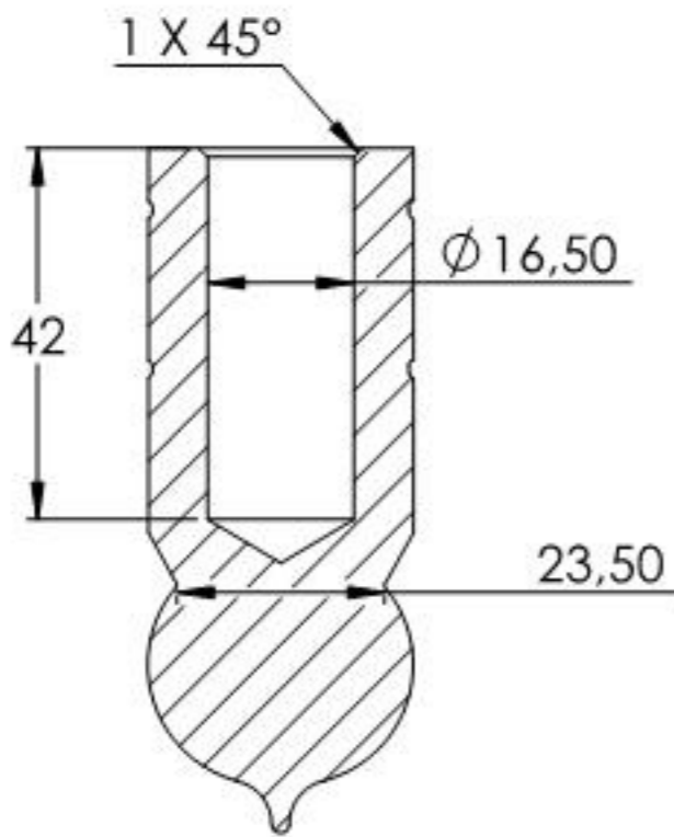
SCHNITT C-C
