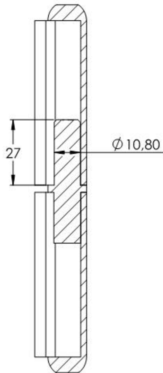
SCHNITT A-A
