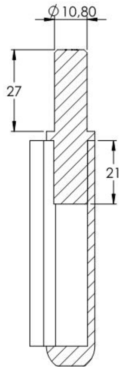
SCHNITT C-C
