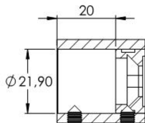
SCHNITT A-A
