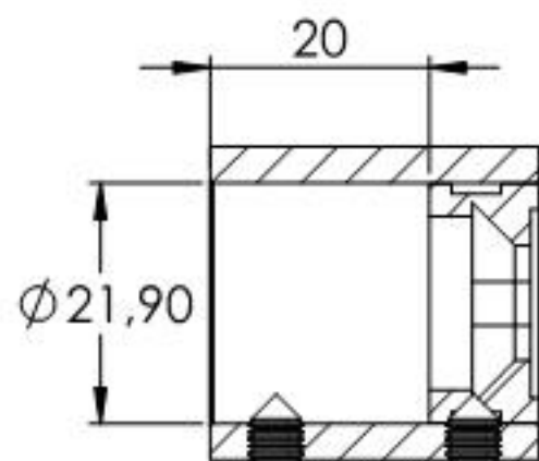
SCHNITT A-A
