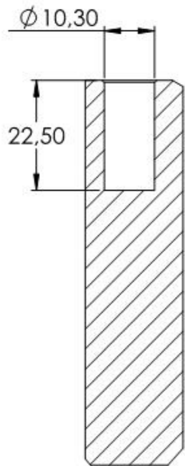
SCHNITT B-B
