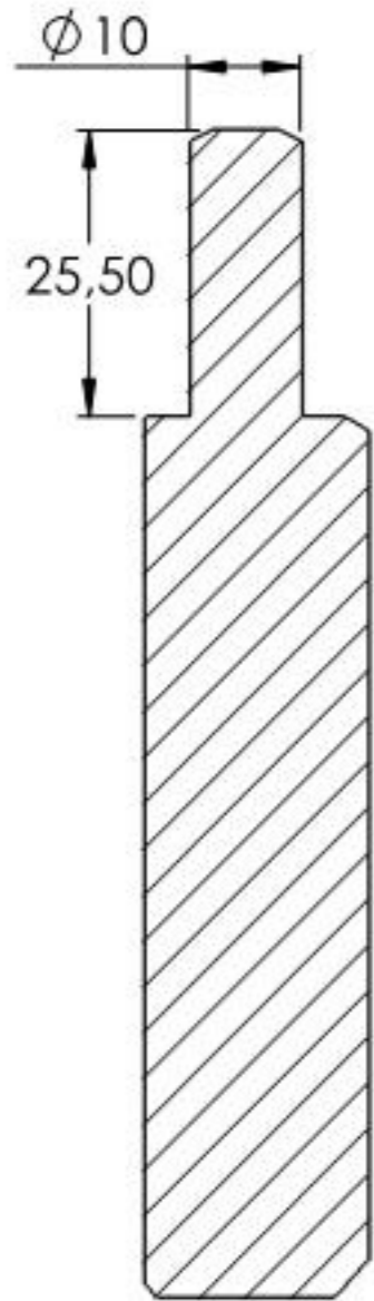
SCHNITT C-C
