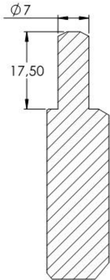
SCHNITT C-C
