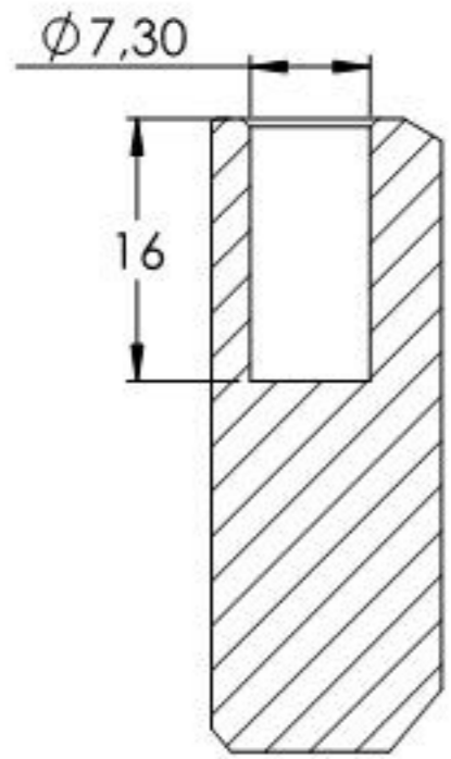
SCHNITT B-B
