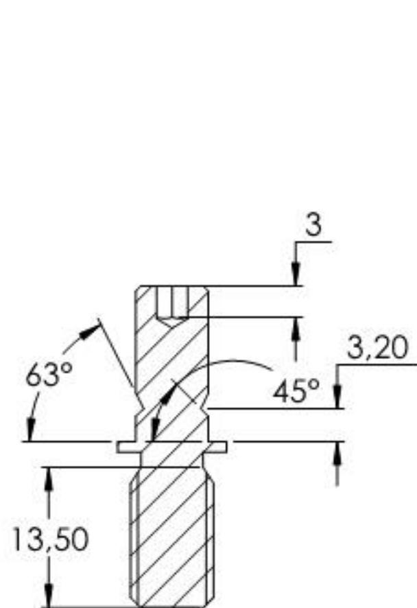
SCHNITT C-C
